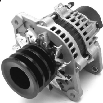
LEA0652 28V / 50A
