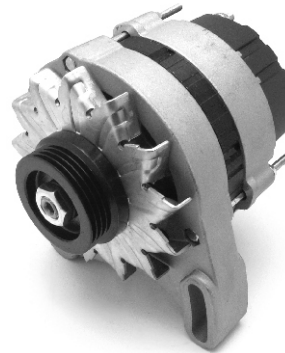
LEA0654 14V / 125A
