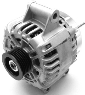
LEA0654 14V / 125A
