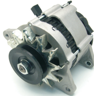
LEA0681 14V / 120A
