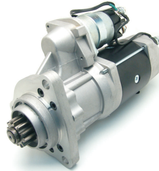
LES0321 24V / 8.3kW
