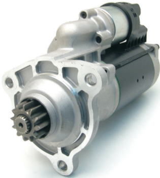
LES0336 24V / 5.5kW
