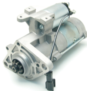
LES0318 24V / 3.2kW
