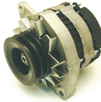
LEA0746 14V / 115A
